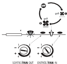
Détail des potentiomètres sur la VRE
