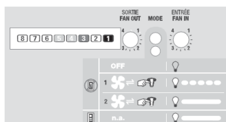
Détail des potentiomètres sur la VRE
