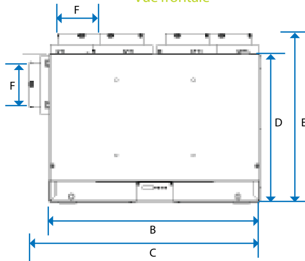
Vue frontale
