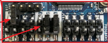
Bornier d'options
